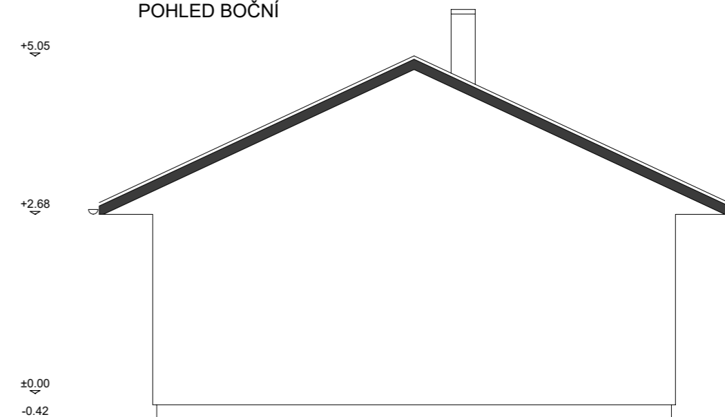
POHLED BOČNÍ
